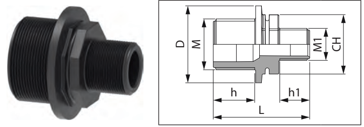
Riduzione maschio/maschio Male/male reducer nipple Reduccion Macho / Macho
