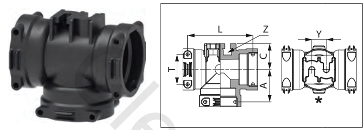
Raccordo a "T" con attacco femmina Tee fitting with female connection Racor en "T" con conexión hembra
