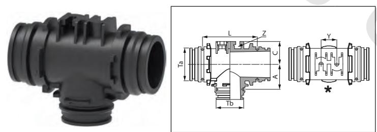
Raccordo a "T" con attacco maschio Tee fitting with male connection Racor en "T" con conexión macho
