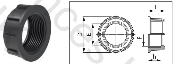
Girello Fly nut Tuerca para racor
