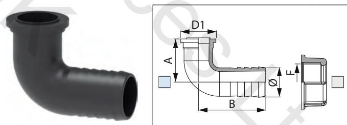
Raccordo portagomma curvo con sede piana per girello 90° hose tail flat seat for fly nut Racor portamanguera curva con asiento plano para tuerca
