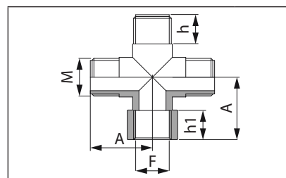
Raccordo filettato a 4 vie 90° maschio/femmina 90°, four-way male/female fitting Rácor de cuatro vías a 90° macho/hembra
