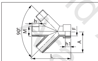
Raccordo filettato a 4 vie 45° maschio/femmina 45°, four-way male/female fitting Rácor de cuatro vías a 45° macho/hembra
