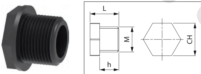
Tappo maschio Male plug Tapón macho
