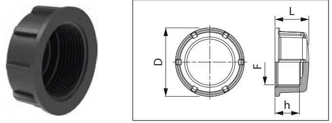
Tappo femmina Blanking cap Tapón hembra
