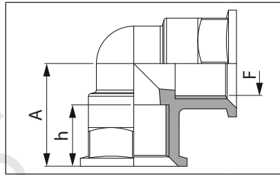
Raccordo filettato curvo 90° femmina/femmina 90° female/female fittings Racor curvo 90° hembra/hembra
