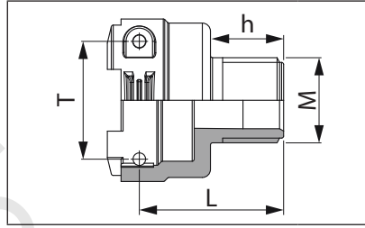
Raccordo filettato maschio attacco femmina Male threaded with female connection Racor roscado macho con conexión hembra
