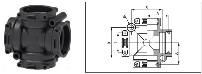
Raccordo 4 vie a 90° con attacco femmina 4-way fitting with female connection Racor de 4 vías a 90° con conexión hembra
