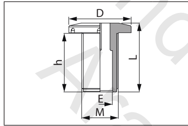
Prese d'acqua antivortice Anti-vortex outlets Conexiones antirremolino
