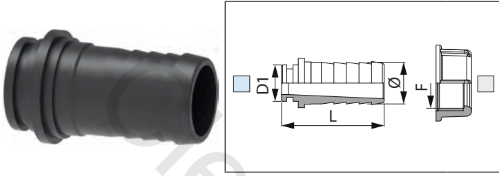
Raccordo portagomma dritto per girello Straight hose fittings for fly nut Racor portamanguera recto para tuerca
