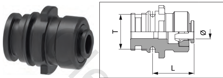
Raccordo dritto maschio per tubo rigido Straight male fitting for rigid pipe Racor recto macho para tubo rígido
