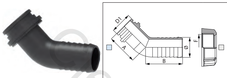
Raccordo portagomma curvo a 45° per girello 45° angled hose fittings for fly nut Racor portamanguera curva a 45° para tuerca
