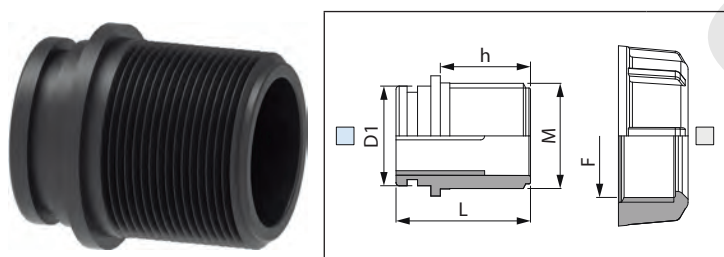
Giunto filettato maschio per girello Coupling with male thread for fly nut Racor roscada macho para tuerca
