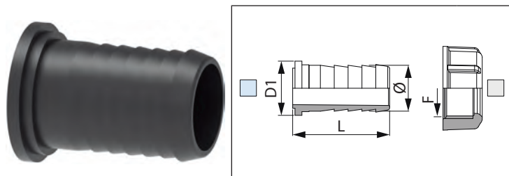
Raccordo portagomma dritto con sede piana per girello Flat seat straight hose tail for fly nut Racor portamanguera recta con asiento plano para tuerca
