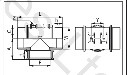
Raccordi a "T" con asole di fissaggio, femmina/maschio Union "Tees" with fastening slots, female/male Rácores en "T" con ranuras de fijación, hembra / macho
