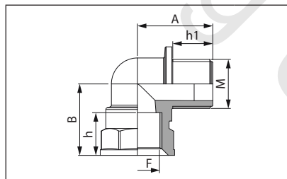
Raccordo filettato curvo 90° maschio/femmina 90° male/female fittings Racor curvo macho/hembra
