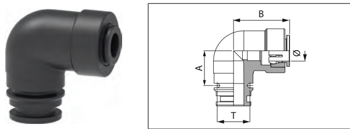
Raccordo curvo maschio per tubo rigido Elbow male fitting for rigid pipe Racor curvo macho para tubo rígido
