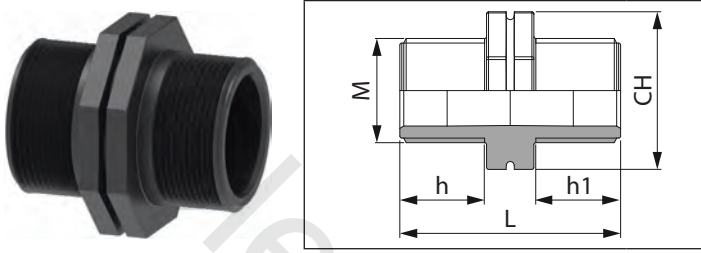
Niplo simmetrico e passaparete Symmetrical and bulkhead nipple Unión simétrico y pasapared
