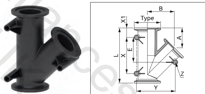
Raccordo Y 3 vie attacco a morsetto* 3-way Y fitting with clamp coupling* Racor Y (3 vías) soporte abrazadera*
